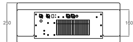
VISTA TRASEIRA
